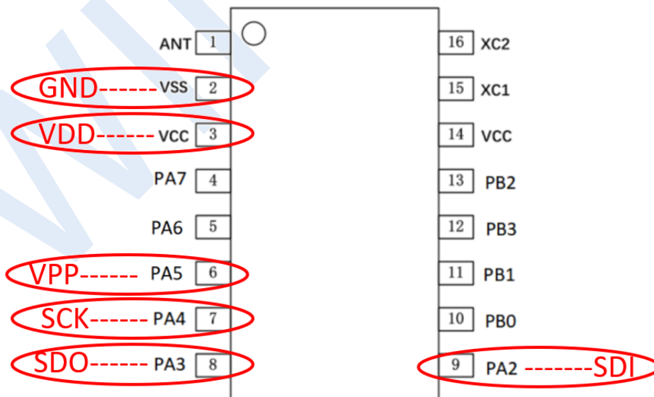
WL2401C烧录脚
